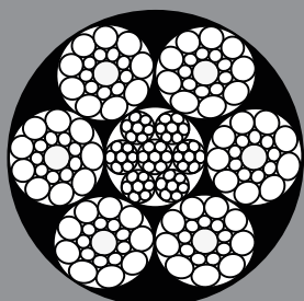
Cabo 6x19 STD Revestido em PVC ou Nylon
