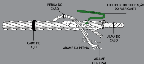
Cabo 6x19 STD Revestido em PVC ou Nylon
