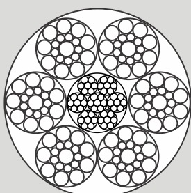
6x19 S
