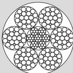
6x25 F
