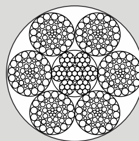
6x41 WS
