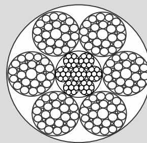
6x29 F
